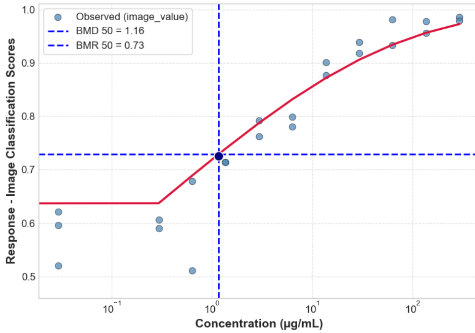
ETOPOSIDE HACAT CTG 24H 4_HACAT_P6_24H_REP1_CTG
