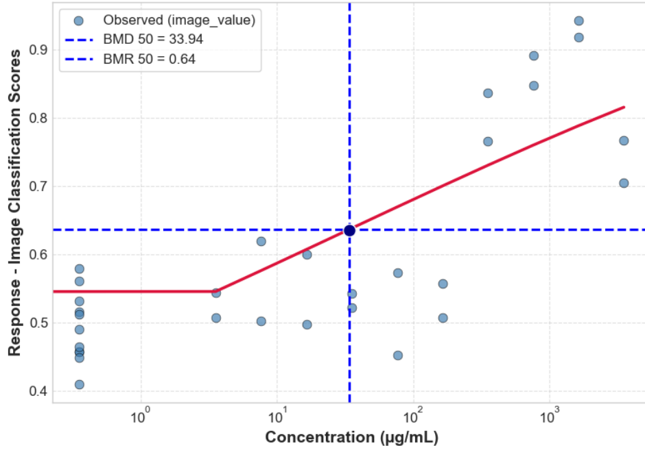
GBF-D HACAT ROSGLO 24H 4_HACAT_P4_24H_REP1_ROSGLO
