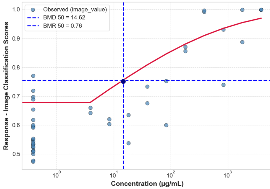
GBF-C HACAT ROSGLO 24H 4_HACAT_P5_24H_REP1_ROSGLO
