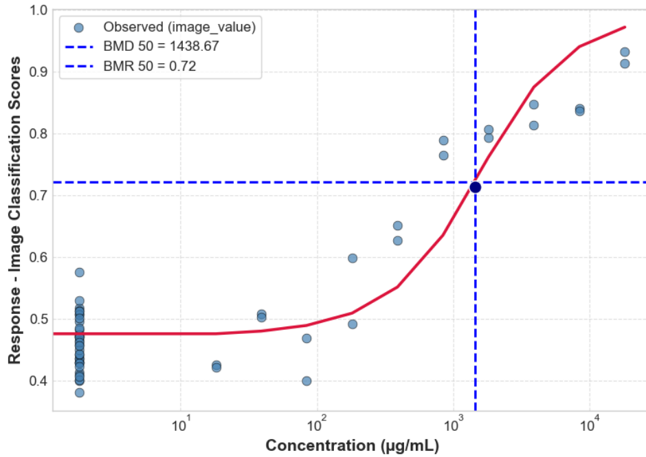
DIQUAT HACAT CTG 24H 4_HACAT_P6_24H_REP2_CTG
