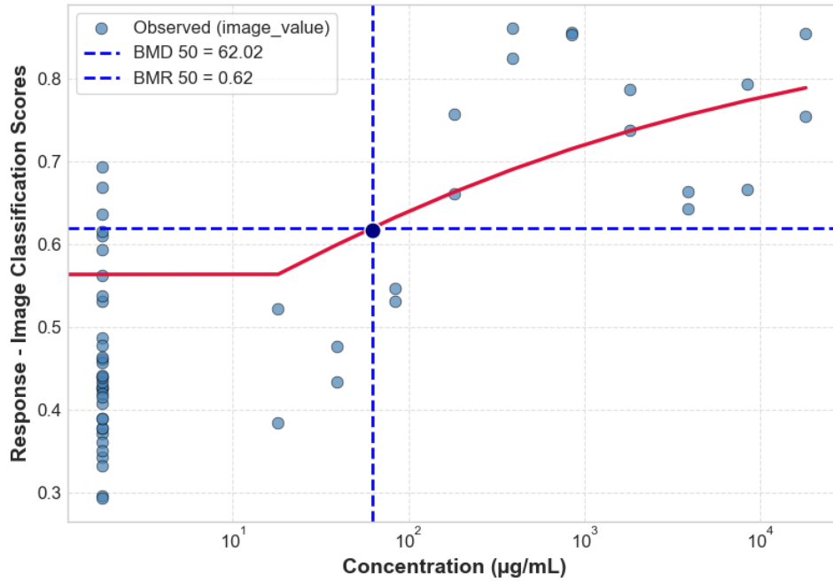
DIQUAT HACAT CTG 24H 4_HACAT_P6_24H_REP6_CTG
