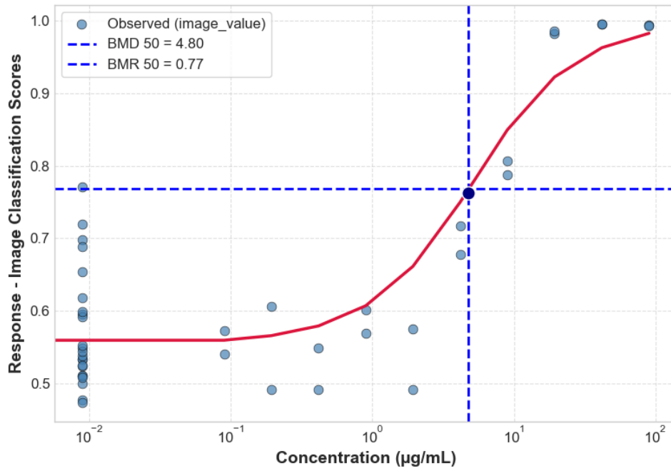
TBHP HACAT ROSGLO 24H 4_HACAT_P5_24H_REP1_ROSGLO
