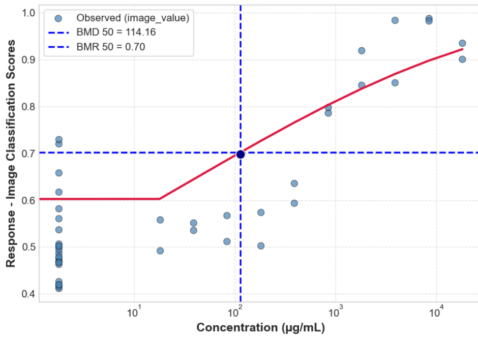
DIQUAT HACAT CTG 24H 4_HACAT_P5_24H_REP2_CTG
