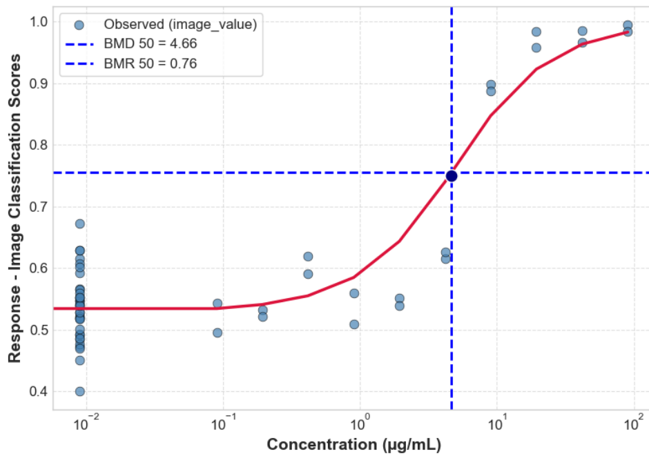
TBHP HACAT CTG 24H 4_HACAT_P6_24H_REP1_CTG
