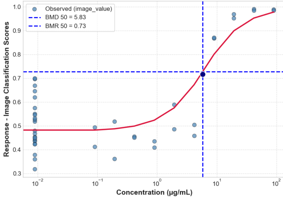
TBHP HACAT ROSGLO 24H 4_HACAT_P5_24HR_REP4_ROS
