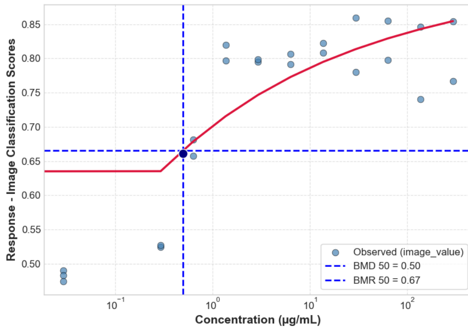
ETOPOSIDE HACAT CTG 24H 4_HACAT_P4_24H_REP2_CTG
