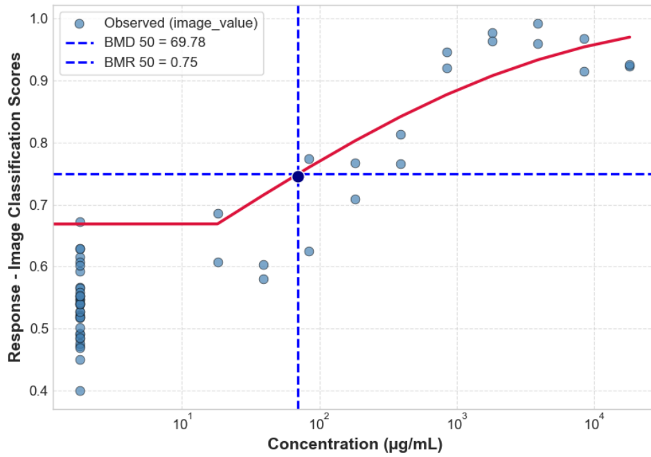
DIQUAT HACAT CTG 24H 4_HACAT_P6_24H_REP1_CTG
