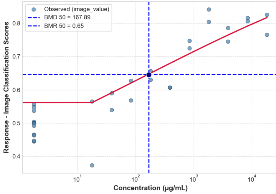
DIQUAT HACAT CTG 24H 4_HACAT_P4_24H_REP2_CTG
