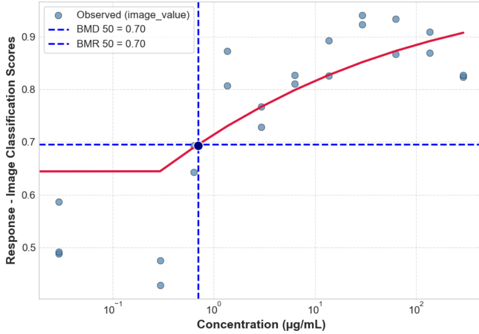
ETOPOSIDE HACAT CTG 24H 4_HACAT_P6_24H_REP2_CTG
