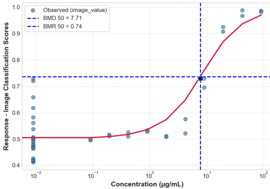
TBHP HACAT CTG 24H 4_HACAT_P5_24H_REP2_CTG
