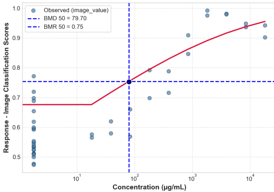
DIQUAT HACAT ROSGLO 24H 4_HACAT_P5_24H_REP1_ROSGLO
