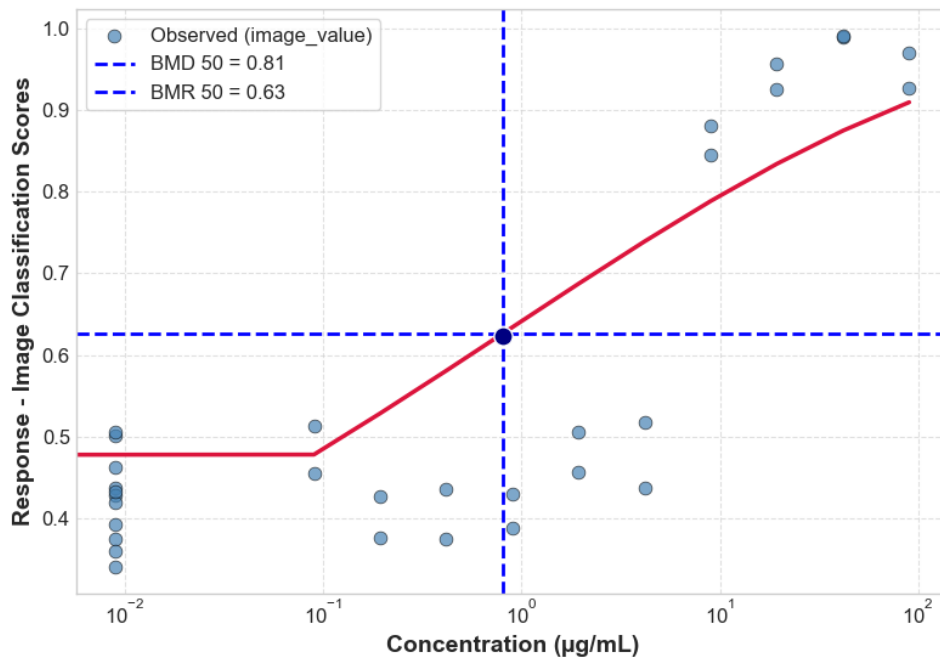
TBHP HACAT ROSGLO 24H 4_HACAT_P4_24HR_REP4_ROS
