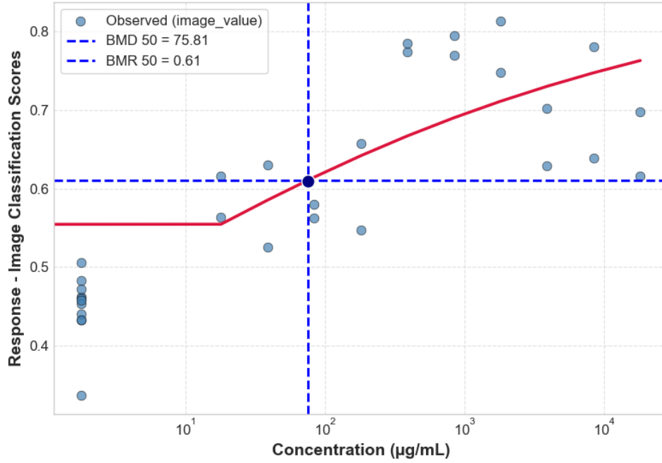
DIQUAT HACAT CTG 24H 4_HACAT_P4_24H_REP6_CTG
