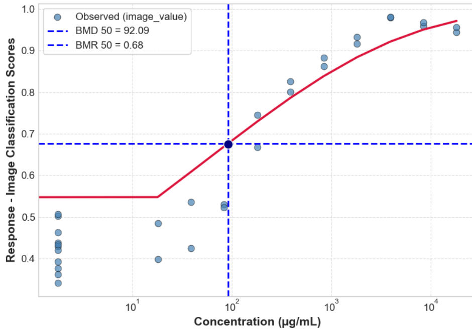
DIQUAT HACAT ROSGLO 24H 4_HACAT_P4_24HR_REP4_ROS
