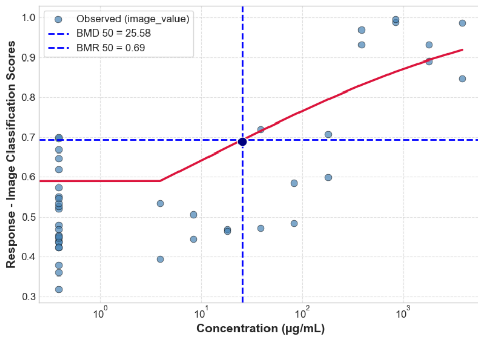
GBF-C HACAT ROSGLO 24H 4_HACAT_P5_24HR_REP4_ROS
