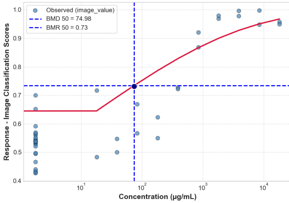
DIQUAT HACAT CTG 24H 4_HACAT_P5_24H_REP1_CTG
