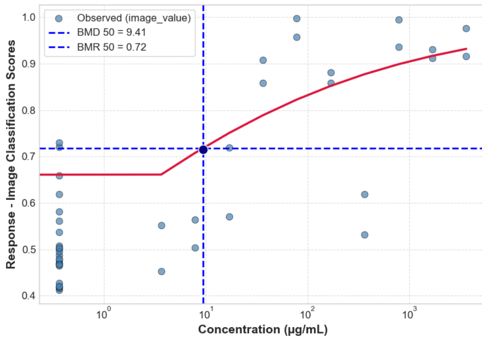
GBF-F HACAT CTG 24H 4_HACAT_P5_24H_REP2_CTG
