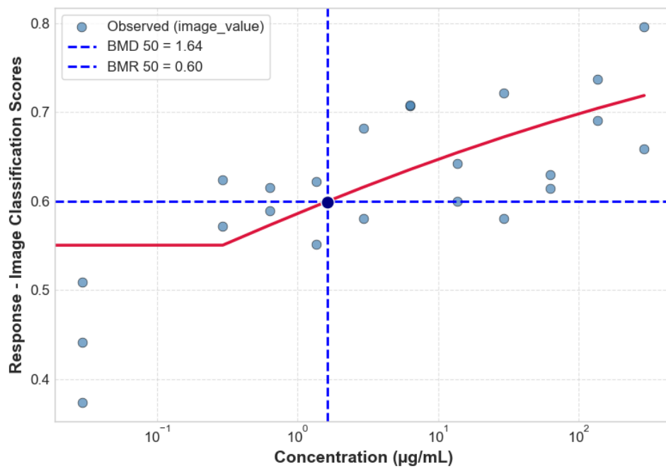
ETOPOSIDE HACAT CTG 24H 4_HACAT_P4_24H_REP6_CTG
