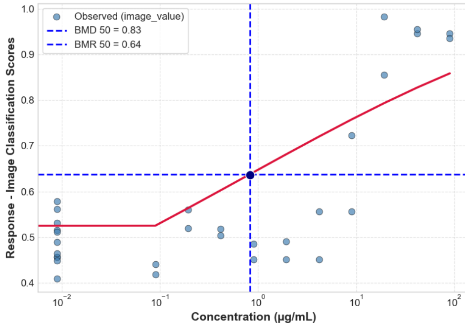
TBHP HACAT ROSGLO 24H 4_HACAT_P4_24H_REP1_ROSGLO
