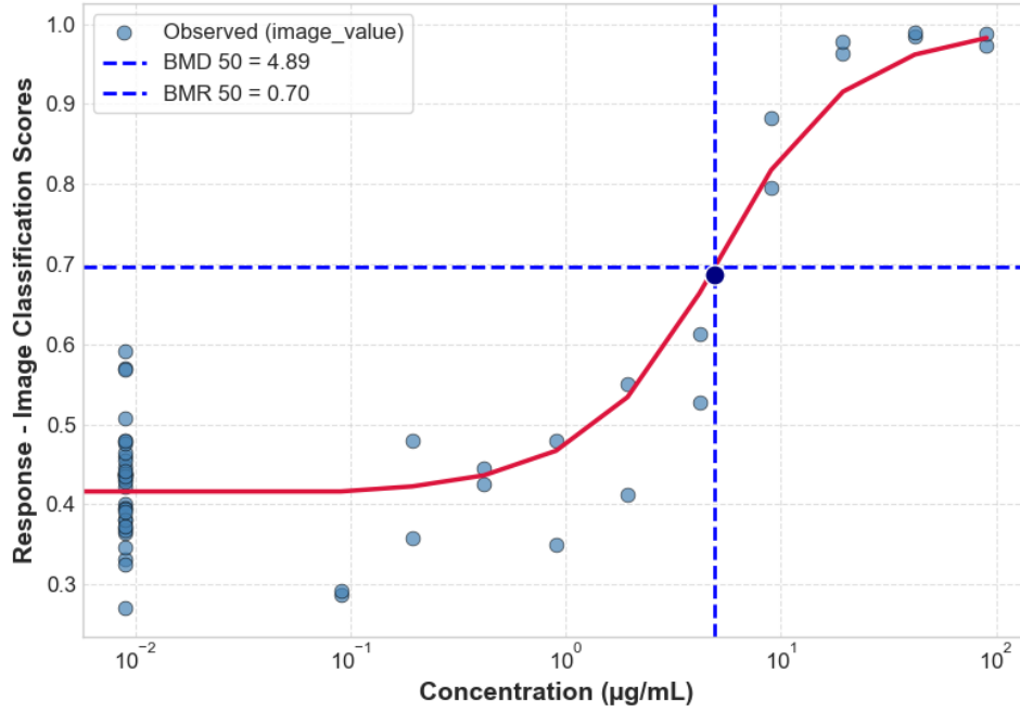
TBHP HACAT ROSGLO 24H 4_HACAT_P6_24HR_REP4_ROS
