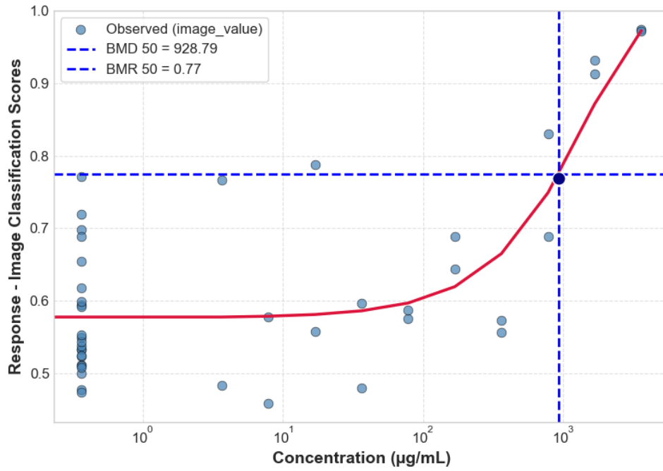
GBF-F HACAT ROSGLO 24H 4_HACAT_P5_24H_REP1_ROSGLO
