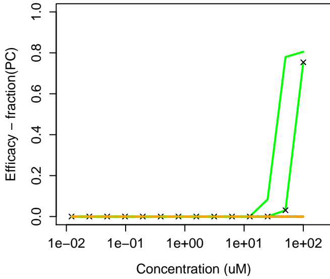
12427-38-2 : Maneb
