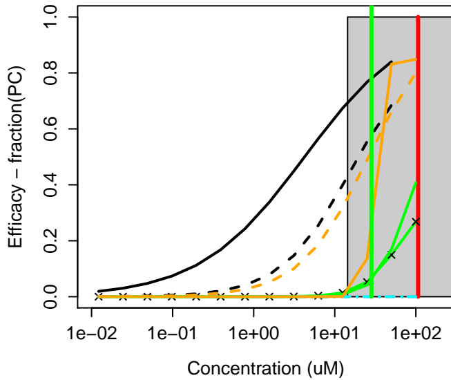
107-54-0 : 3,5-Dimethyl-1-hexyn-3-ol
