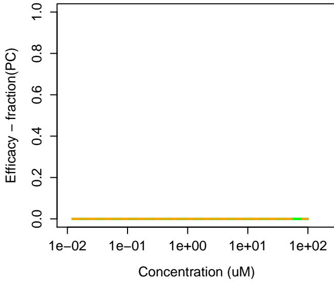
100-54-9 : 3-Pyridinecarbonitrile
