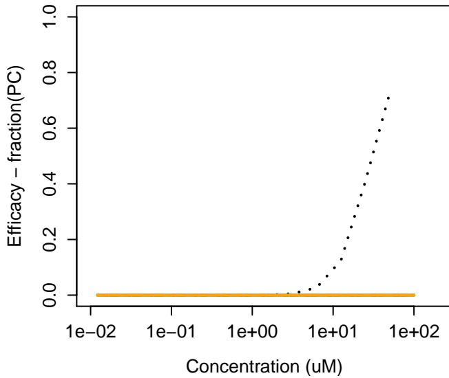
86-30-6 : N-Nitrosodiphenylamine
