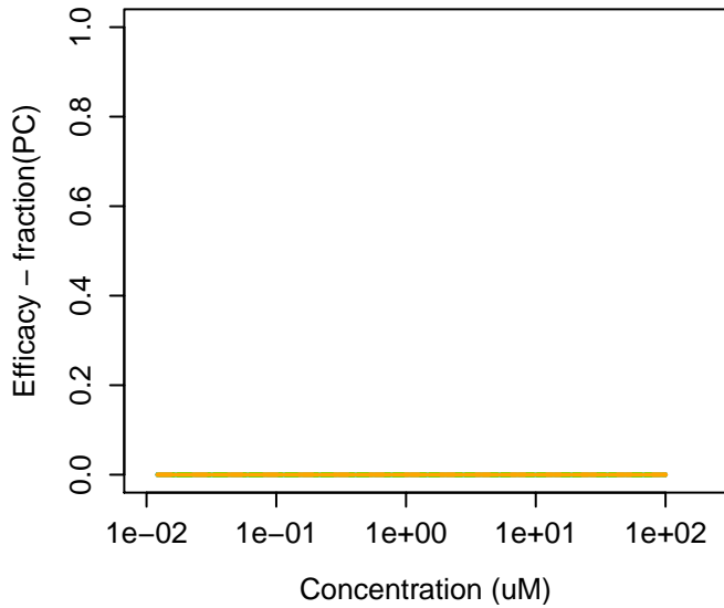
189003-92-7 : Trelanserin
