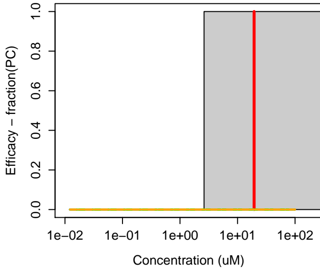
83-32-9 : Acenaphthene
