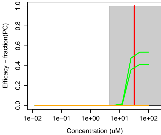
8018-01-7 : Mancozeb
