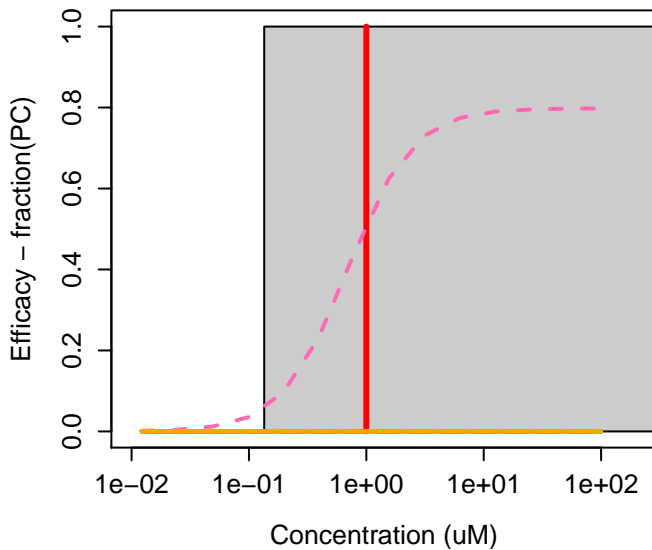
100-64-1 : Cyclohexanone oxime
