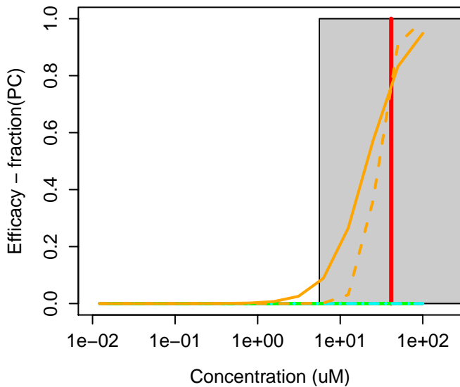
68157-60-8 : Forchlorfenuron
