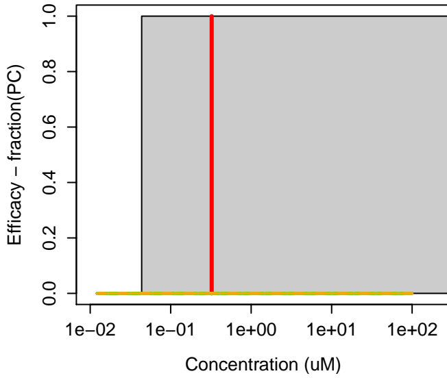
111-76-2 : 2-Butoxyethanol
