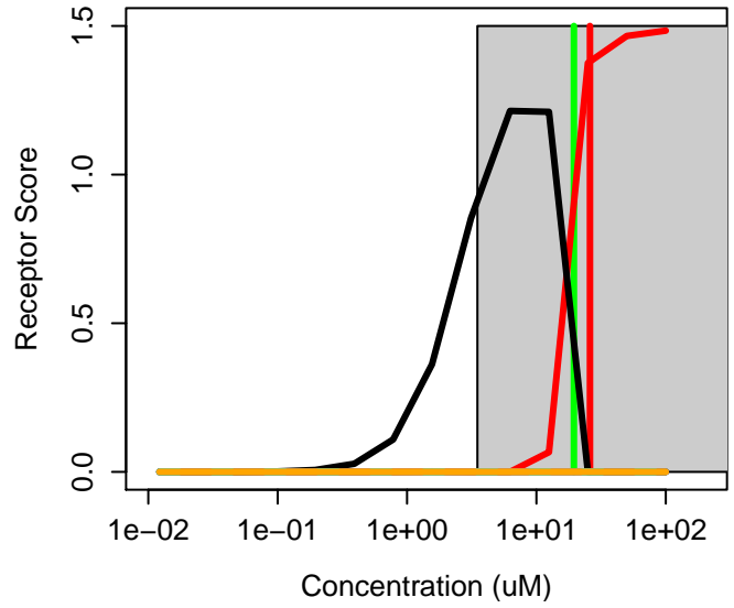
6846-50-0 : 2,2,4-Trimethyl-1,3-pentanediol diisobu 6846-50-0 : 2,2,4-Trimethyl-1,3-pentanediol diisobu Agonist: 0 Antagonist: 0
