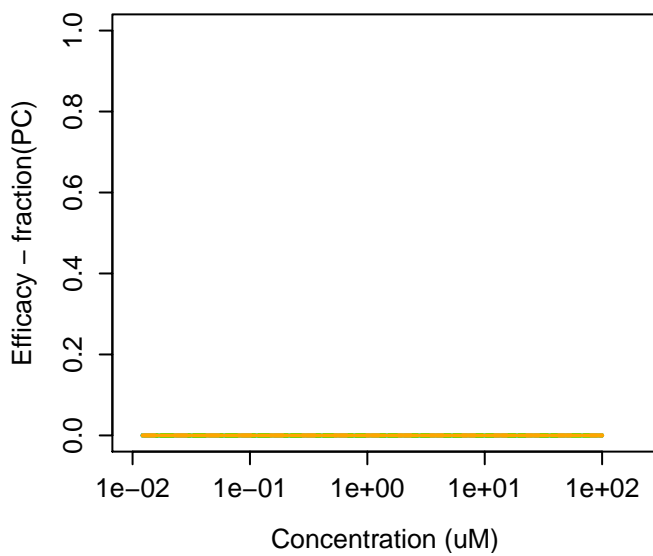
94-82-6 : 2,4-DB
