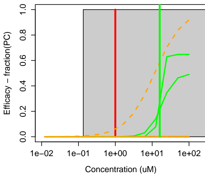
705-60-2 : (2-Nitro-1-propenyl)benzene
