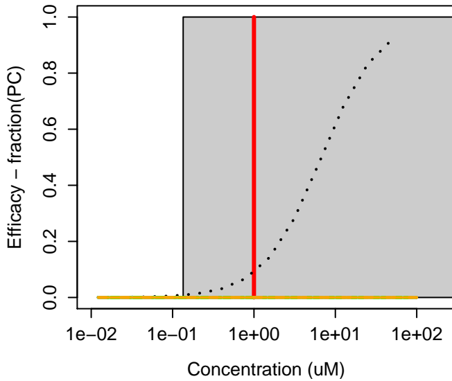
9004-96-0 : Polyoxyethylene monoleate
