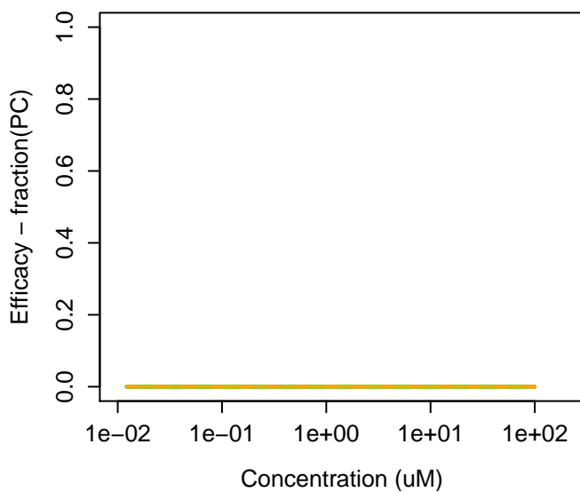
16672-87-0 : Ethephon
