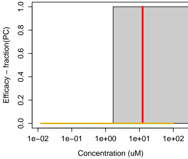
98-01-1 : Furfural
