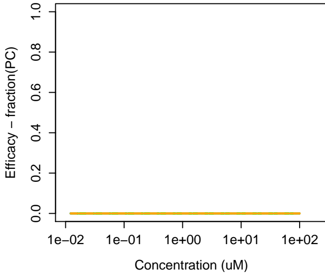
1634-78-2 : Malaoxon
