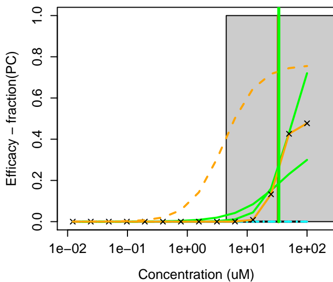
1836-75-5 : Nitrofen
