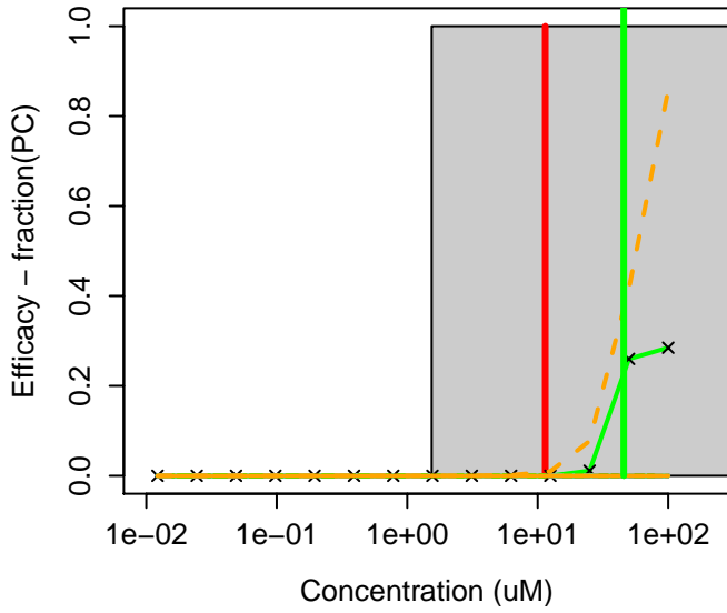
78-59-1 : Isophorone
