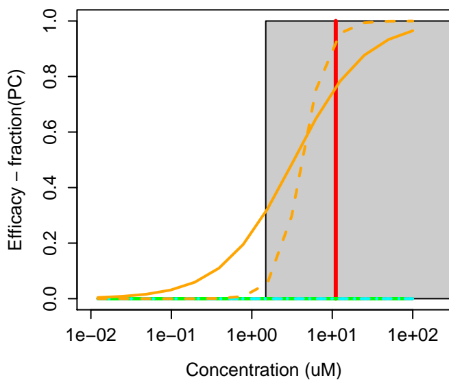
249296-43-3 : CJ-013610
