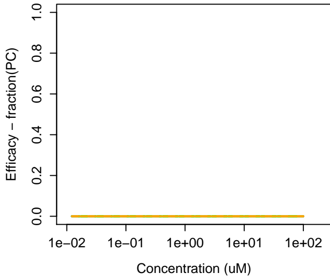
20830-75-5 : Digoxin
