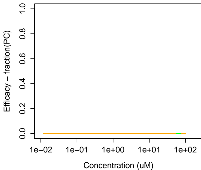
98-54-4 : 4-tert-Butylphenol
