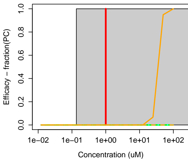
491-80-5 : Biochanin A
