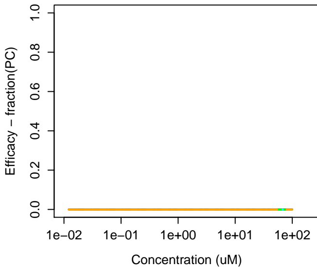
94-13-3 : Propylparaben
