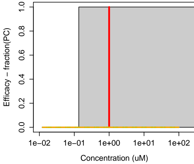
97-53-0 : Eugenol
