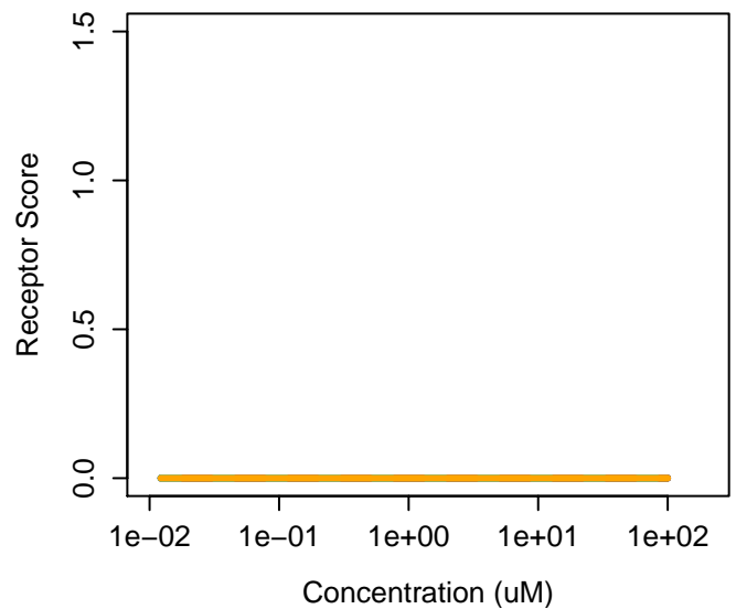
14233-37-5 : 1,4-Bis(N-isopropylamino)anthraquin 14233-37-5 : 1,4-Bis(N-isopropylamino)anthraquin Agonist: 0 Antagonist: 0
