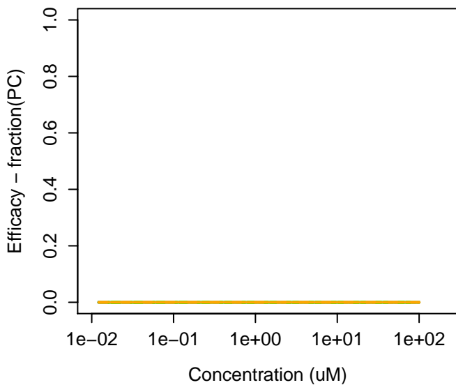
124378-77-4 : Enadoline
