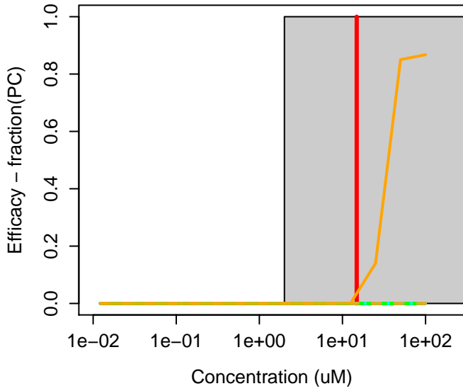
1134-23-2 : Cycloate
