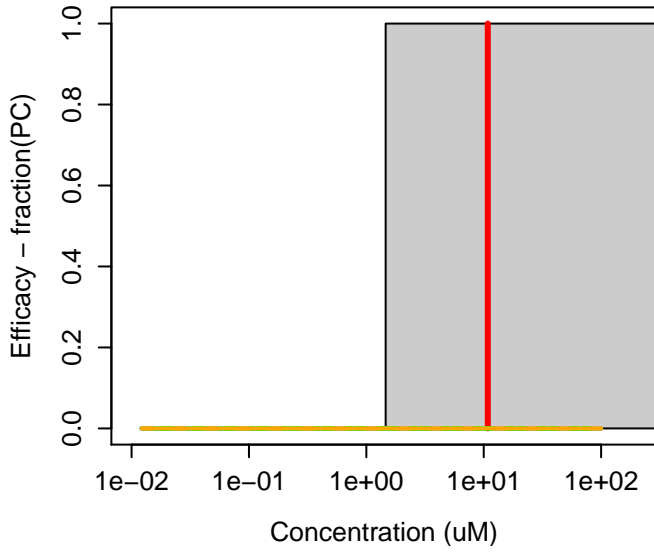
79-57-2 : Oxytetracycline
