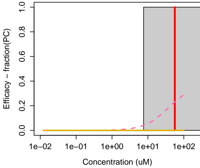
79-24-3 : Nitroethane
