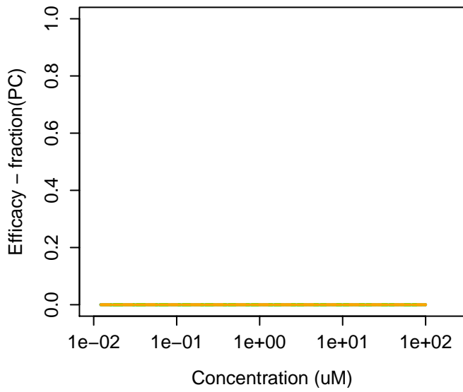
75-99-0 : Dalapon
