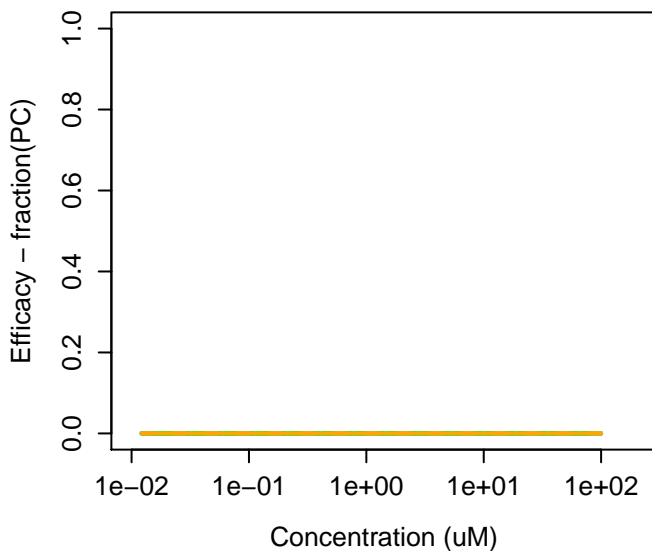
107-87-9 : 2-Pentanone
