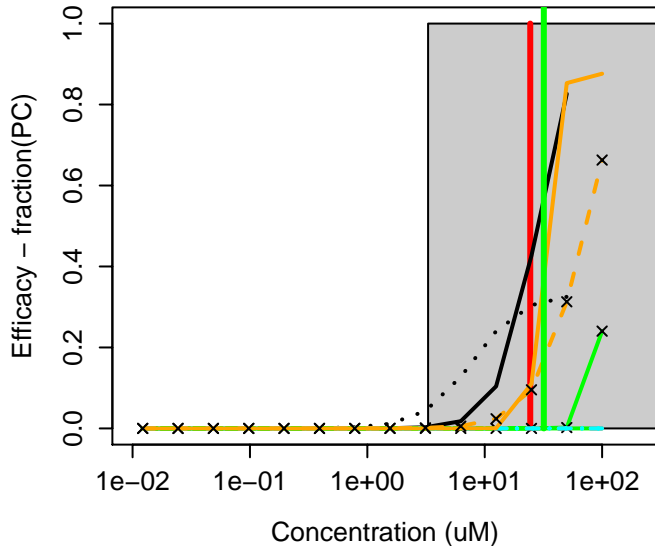
58-89-9 : Lindane
