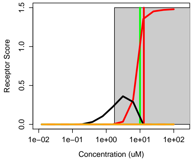
97-23-4 : Dichlorophen Agonist: 0 Antagonist: 0.34
