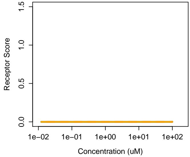
: 4-(2-Phenylpropan-2-yl)-N-[4-(2-phenylpropan-2-yl)-N-[4-(2-phenylpropan-2-yl)-N-[4-(2-phenylpropan-2-yl)-N-[4-(2-phenylpropan-2-yl)-N]-N]-N]-N]-N]-N]-N- Agonist: 0 Antagonist: 0
