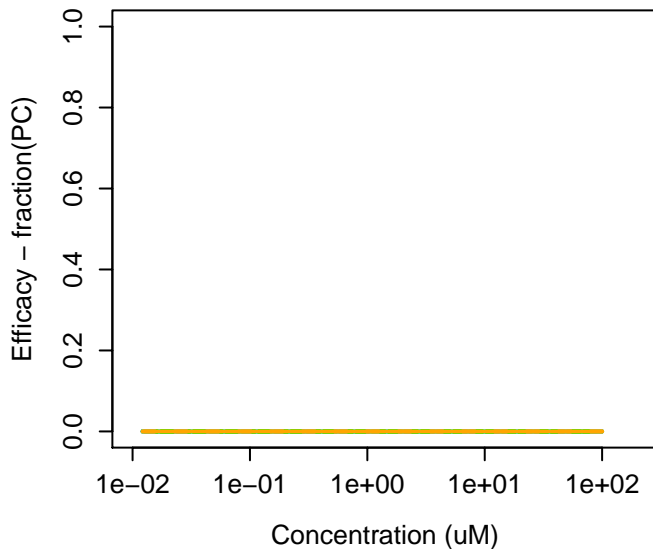
138-22-7 : Butyl lactate
