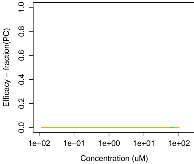
98-06-6 : tert-Butylbenzene
