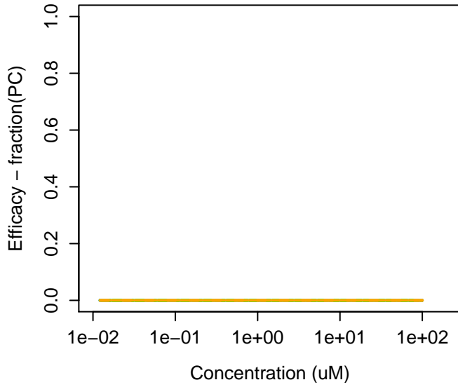
118134-30-8 : Spiroxamine
