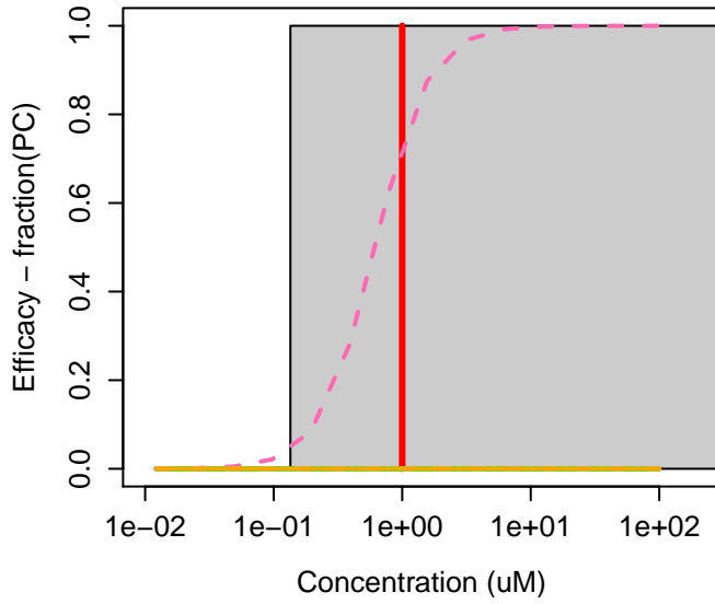
112-34-5 : 2-(2-Butoxyethoxy)ethanol
