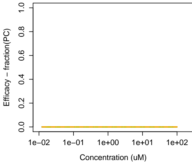
108-95-2 : Phenol
