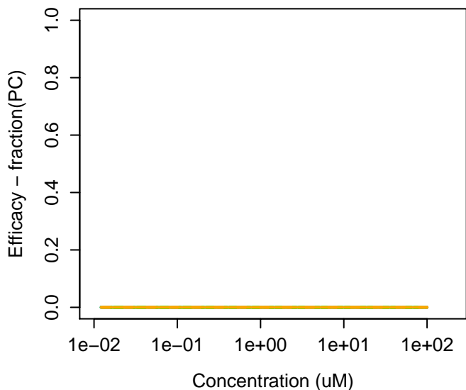
55589-62-3 : Acesulfame potassium
