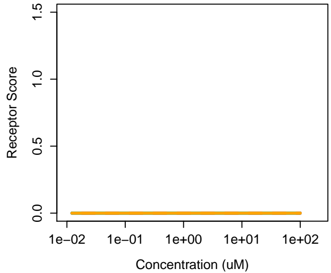
189003-92-7 : Trelanserin Agonist: 0 Antagonist: 0.029
