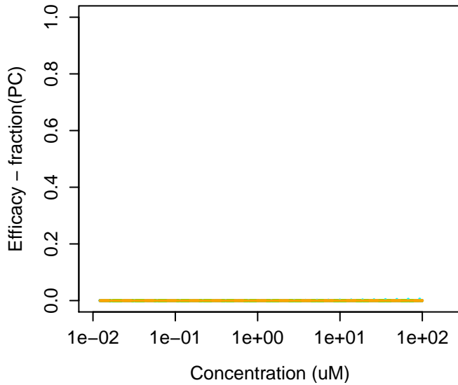
14233-37-5 : 1,4-Bis(N-isopropylamino)anthraquin 14233-37-5 : 1,4-Bis(N-isopropylamino)anthraquin Agonist: 0 Antagonist: 0
