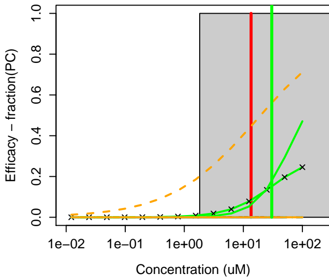
40487-42-1 : Pendimethalin
