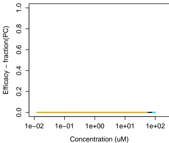
17465-86-0 : gamma-Cyclodextrin
