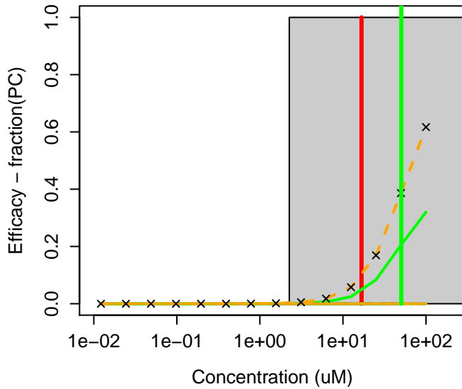
55285-14-8 : Carbosulfan
