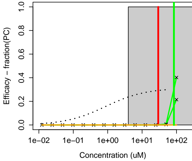
23089-26-1 : Levomenol
