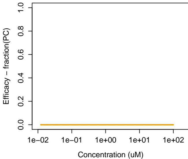
102-82-9 : Tributylamine
