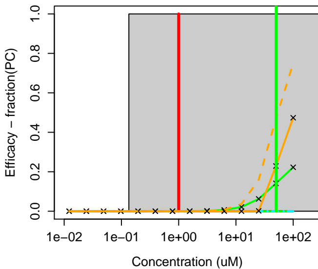
959-98-8 : Endosulfan I
