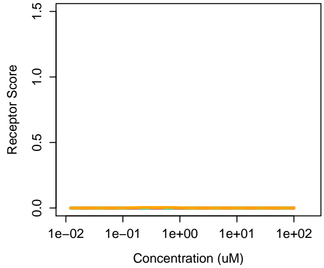
21087-64-9 : Metribuzin Agonist: 0 Antagonist: 0
