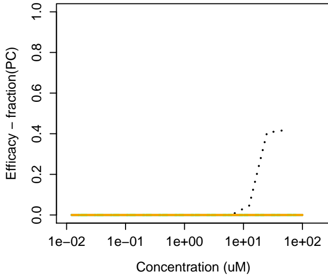
: 4-(2-Phenylpropan-2-yl)-N-[4-(2-phenylpropan-2-yl)-N-[4-(2-phenylpropan-2-yl)-N-[4-(2-phenylpropan-2-yl)-N-[4-(2-phenylpropan-2-yl)-N]-N]-N]-N]-N]-N]-N- Agonist: 0 Antagonist: 0
