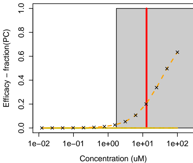
129-00-0 : Pyrene
