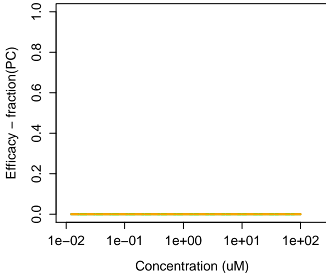
129-17-9 : Sulfan blue
