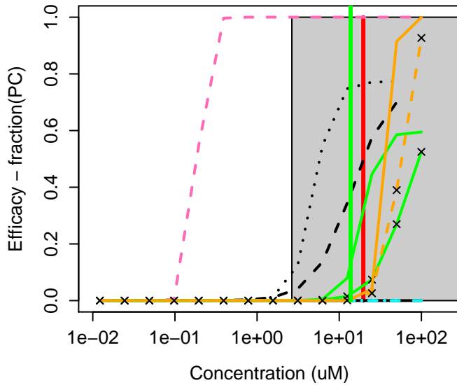
19780-11-1 : (2-Dodeceny)succinic anhydride
