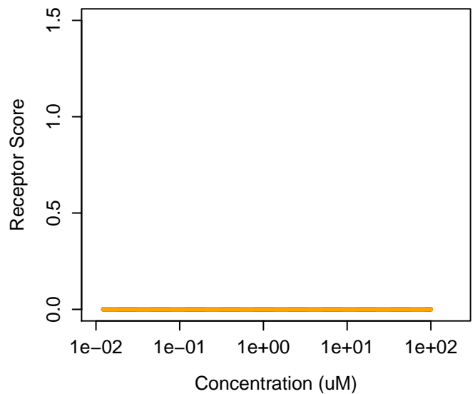
1008-72-6 : Sodium 2-formylbenzenesulfonate Agonist: 0 Antagonist: 0
