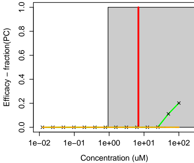
118-47-8 : Pyrazolone T
