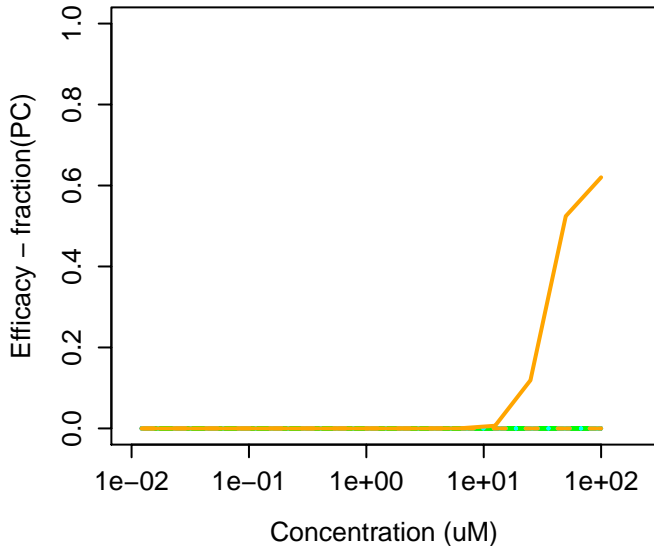
402910-27-4 : UK-416244
