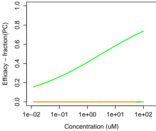
119-61-9 : Benzophenone
