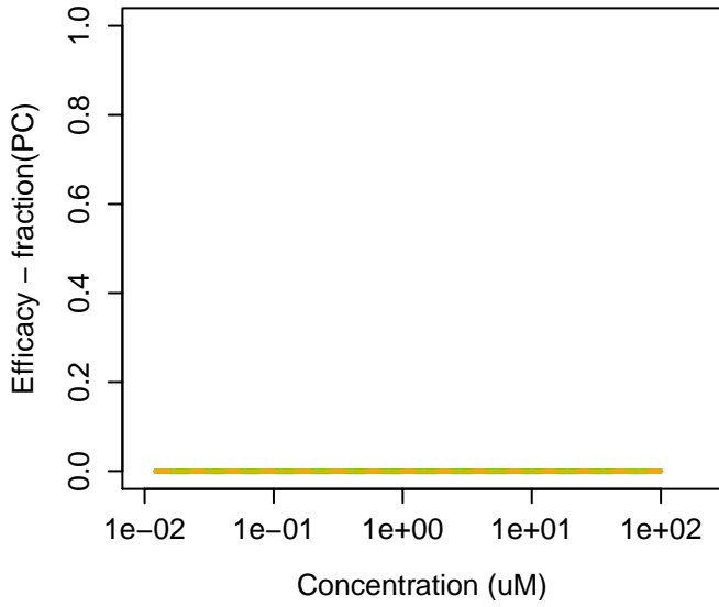
: 1-(6-tert-Butyl-1,1-dimethyl-2,3-dihydro-1H-indol-3-yl)ethan-1-one : 1-(6-tert-Butyl-1,1-dimethyl-2,3-dihydro-1H-indol-3-yl)ethan-1-one Agonist: 6e-05 Antagonist: 0
