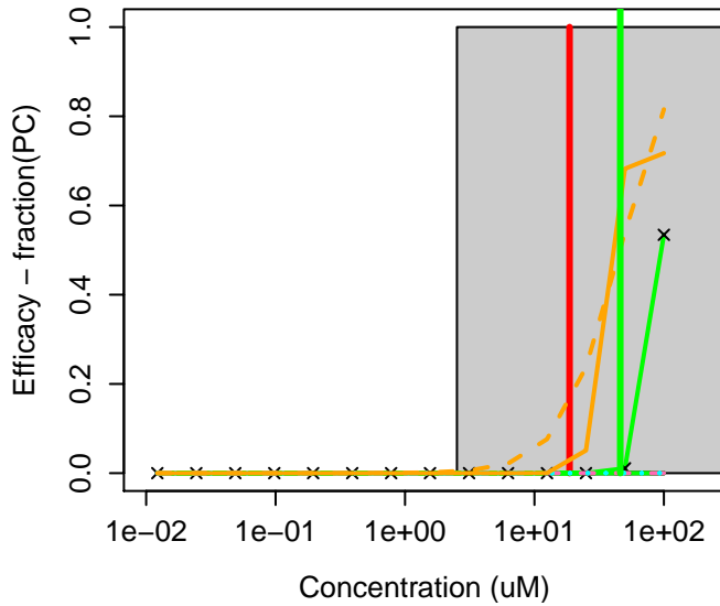
124-68-5 : 2-Amino-2-methylpropan-1-ol
