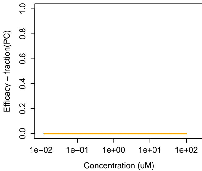
70-55-3 : 4-Toluenesulfonamide
