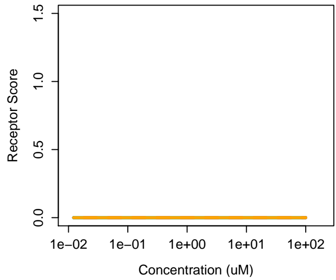
118-71-8 : Maltol Agonist: 0 Antagonist: 0
