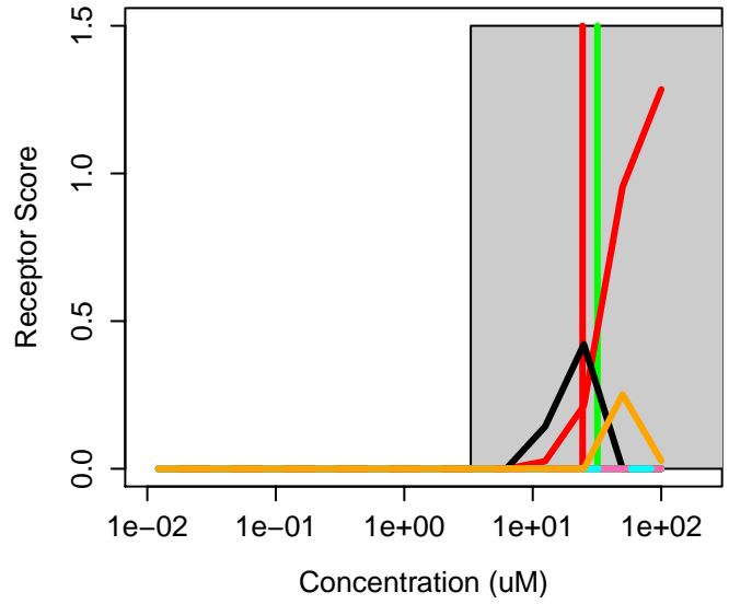
58-89-9 : Lindane Agonist: 0 Antagonist: 0
