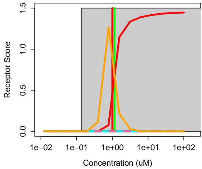
4344-55-2 : 4-Butyloxyaniline Agonist: 0 Antagonist: 0
