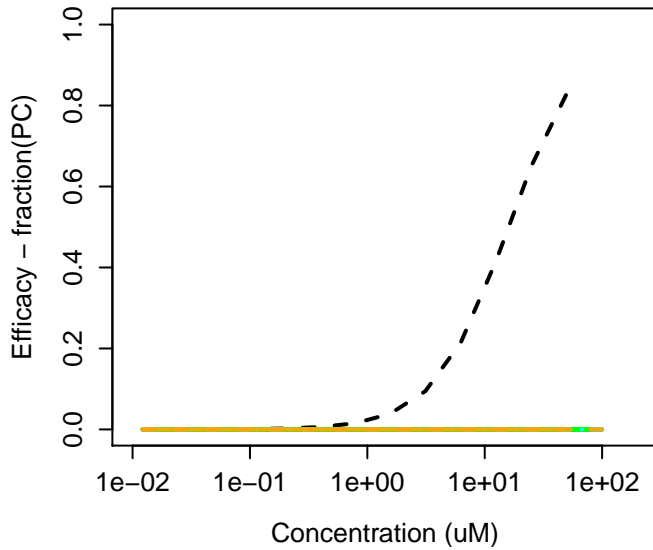
616-45-5 : 2-Pyrrolidinone
