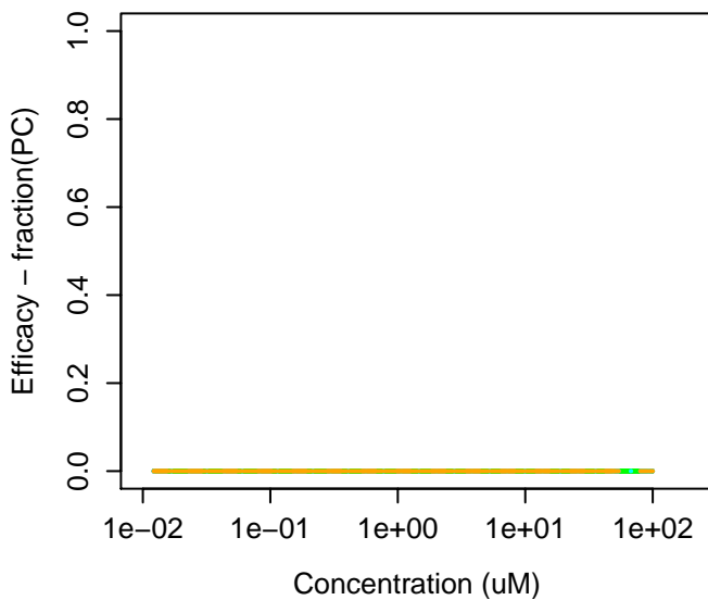
124-04-9 : Hexanedioic acid
