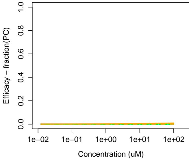
121552-61-2 : Cyprodinil
