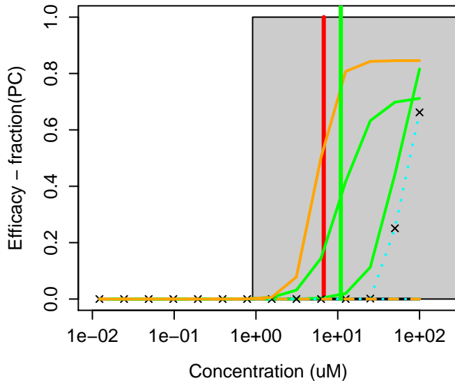
22224-92-6 : Fenamiphos
