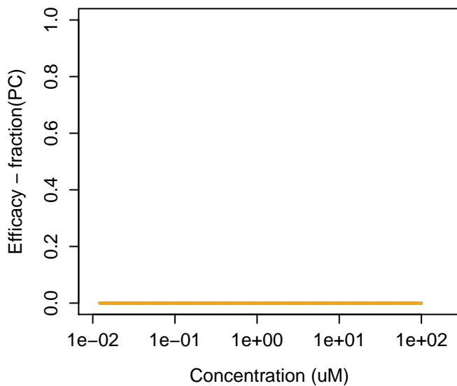
114-26-1 : Propoxur
