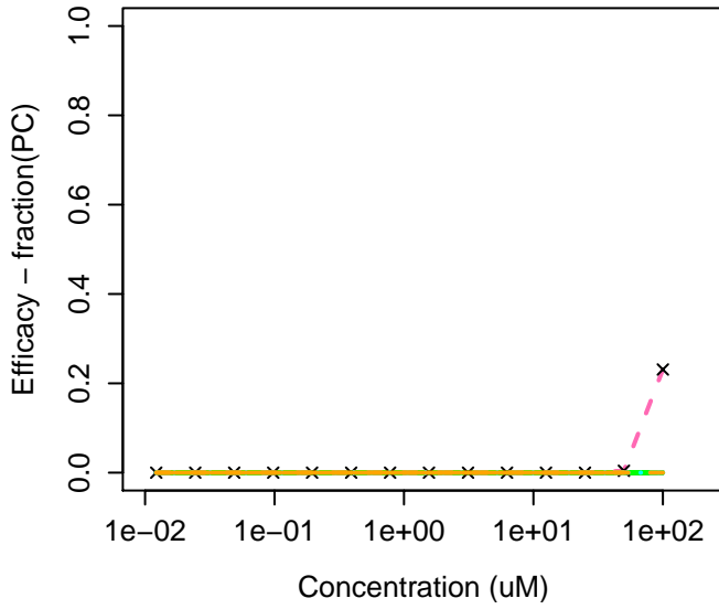
102-76-1 : Triacetin
