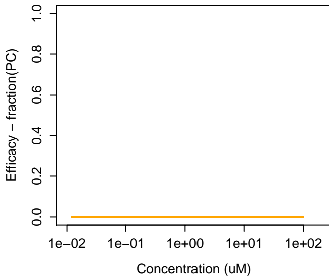
78-70-6 : Linalool
