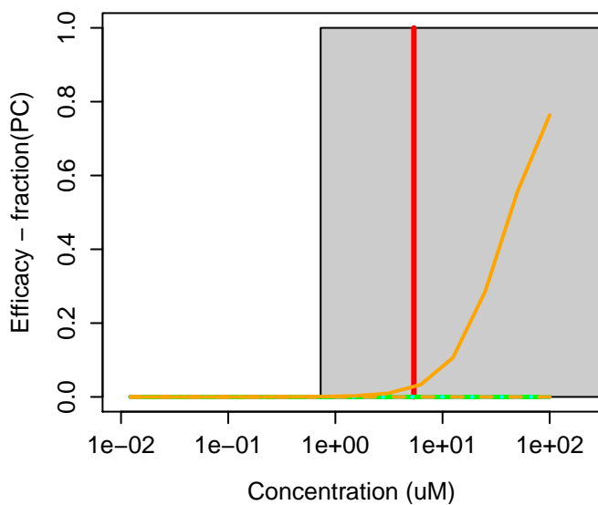
219790-72-4 : SB281832
