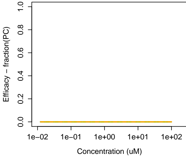
123-99-9 : Nonanedioic acid
