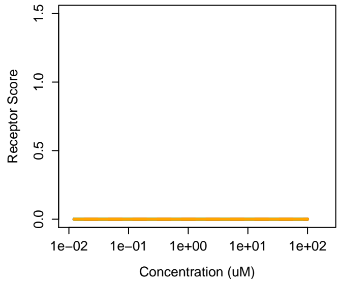
77-73-6 : Dicyclopentadiene Agonist: 0 Antagonist: 0
