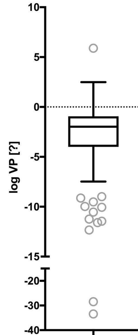
vapour pressure (VP)
